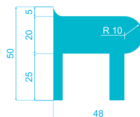
NAROŻNIK ZEWNĘTRZNY MINI
