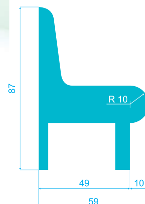
NAROŻNIK KLASYCZNY ZEWNĘTRZNY
